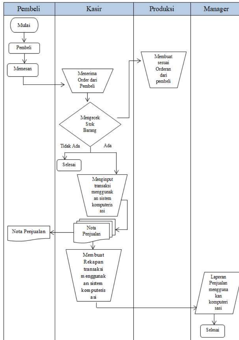
Gambar 4. Usulan Sistem Penjualan Restoran Sop Ikan Batam
